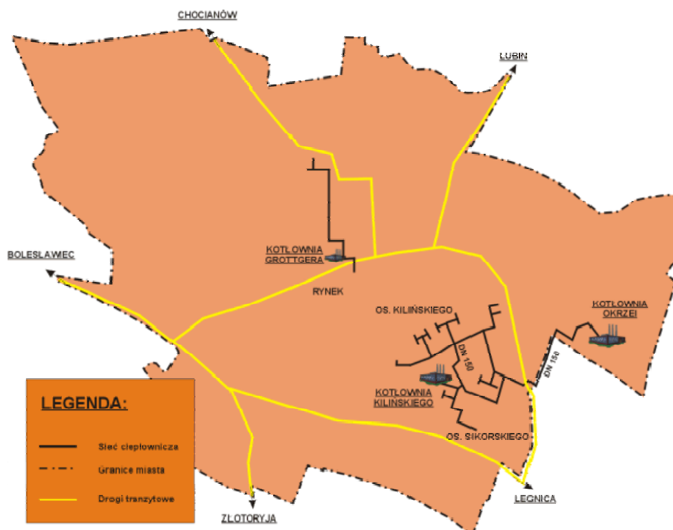
Rysunek 19. System sieci ciepłych i źródeł ciepła WPEC w Legnicy S.A. w mieście Chojnow - stan istniejący
